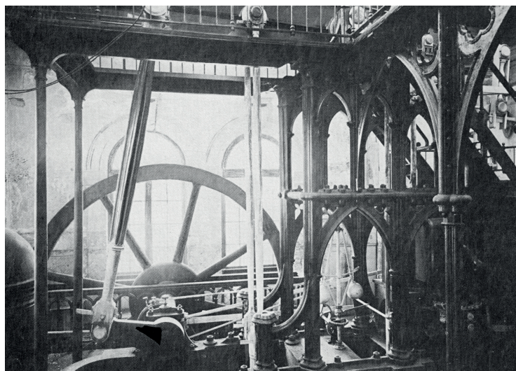
▲ Stoommachine in het eerste pompstation te Leyduin, gebouwd in 1852 (foto 1895).
