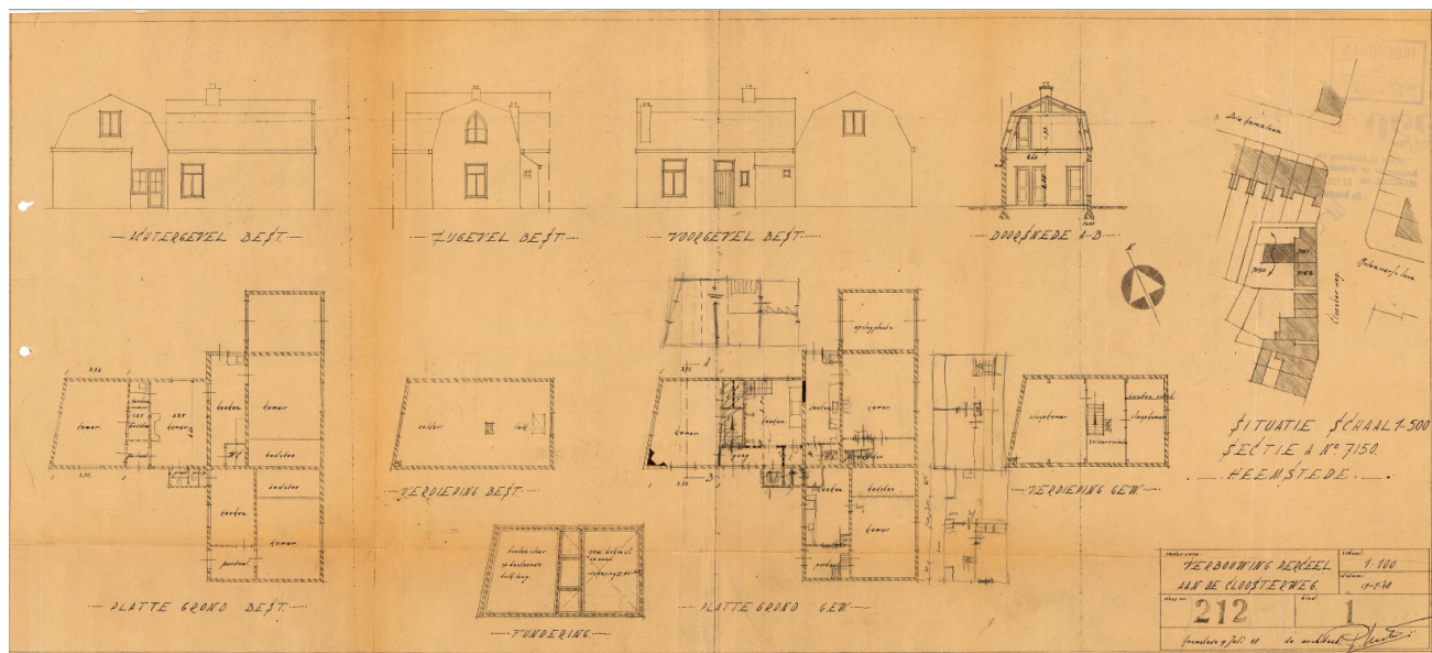
Bouwtekening van 1949 voor Cloosterweg 9
