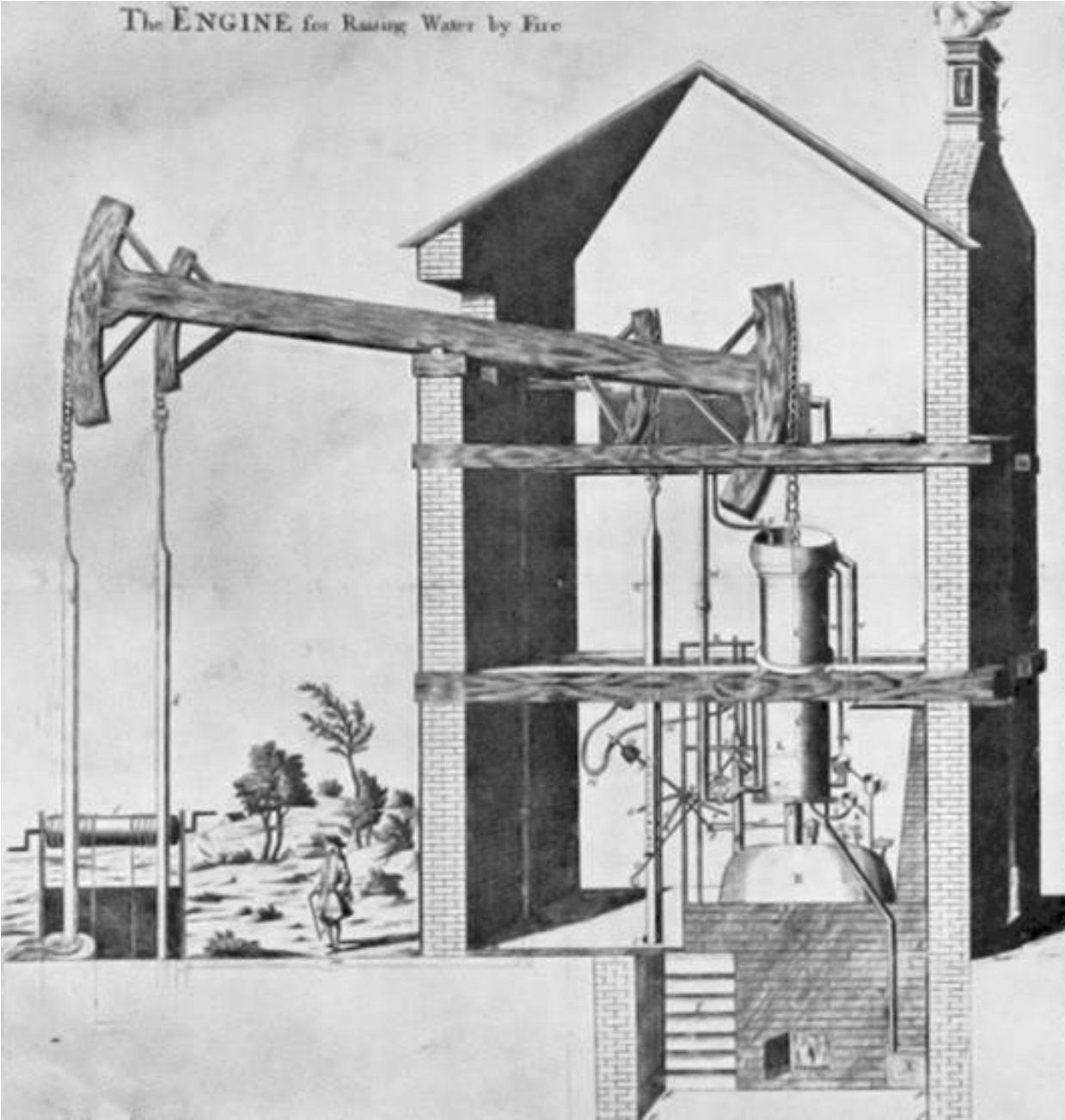
Stoommachine
