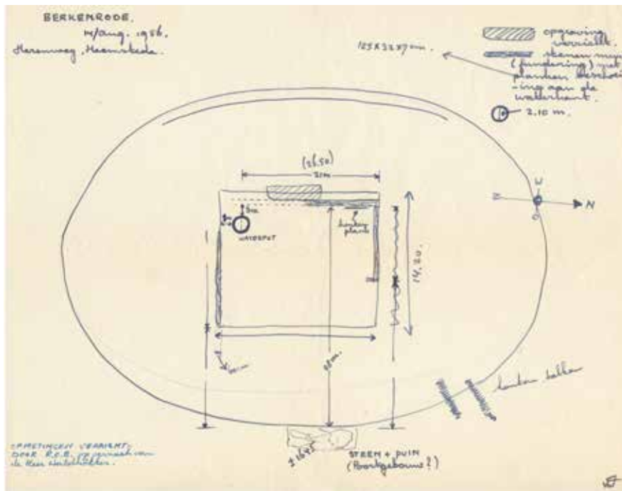
▲ In het midden van de vijver liggen de fundamente van het kasteel Berkenrode. De opgravingen gebeurden aan de westkant van het voormalige kasteel (zie arcering). Tekening Kees Wijdooge, 1956.
