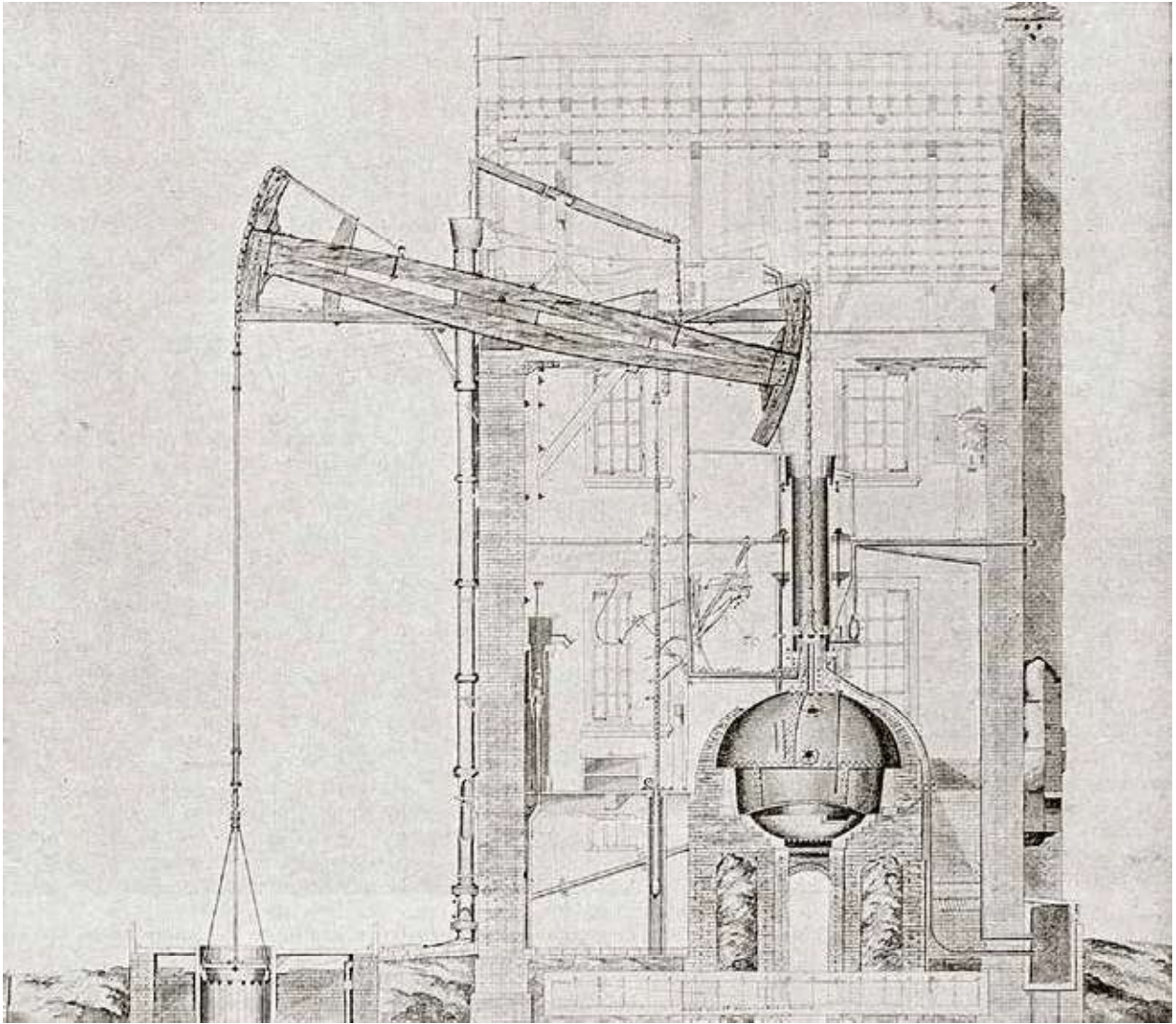
▲ Doorsneetekening van de vuurmachine in Groenendaal, vervaardigd door Rhijnse Lieve Brouwer.
