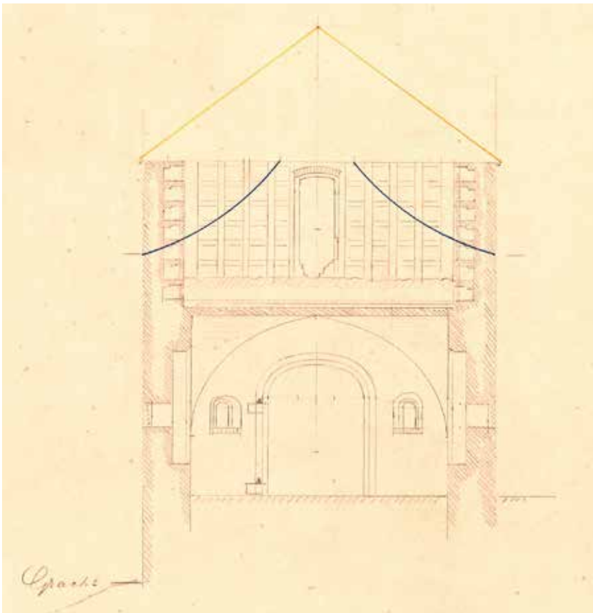
▲ Doorsnedetekening van de Rijkscommissie voor de Monumentenbeschrijving van de bestaande toestand in april 1907.
