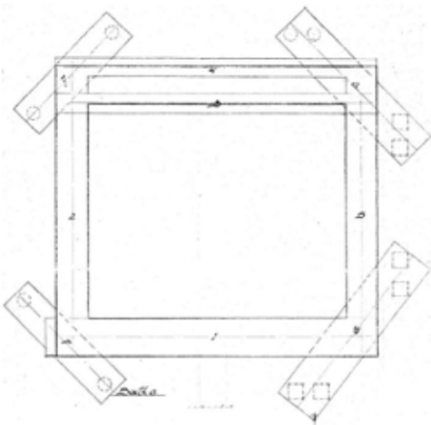
▲ Tekening van de fundering van de duivenpoort uit 1965, volgens hetzelfde uitgangspunt als in 1958. In 1966 werd alles nog eens zorgvuldig nagerekend door een adviesbureau voor bouwkundige constructies.
